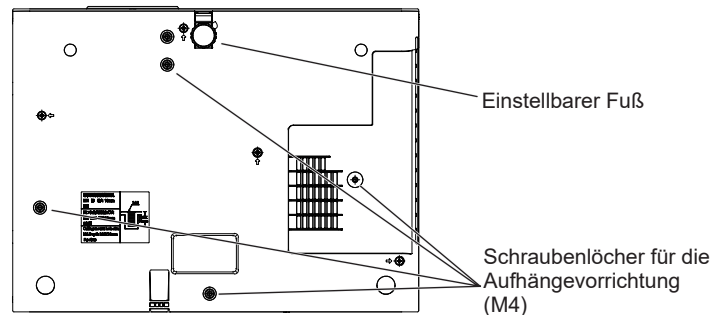
Positionen der Schraubenlöcher für die Aufhängevorrichtung und der einstellbaren Fuß
